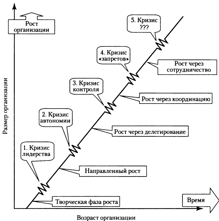
Рис. 14.2. Модель Грейнера
