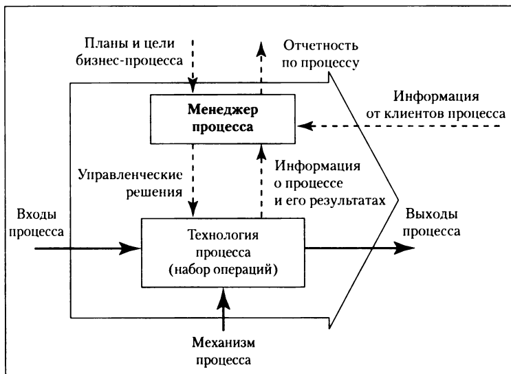
Рис. 7.1. Схема бизнес-процесса
